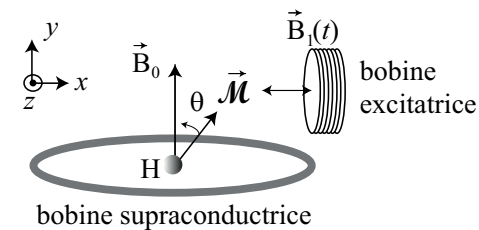
FIGURE 7 – Principe de la RMN et bobines supra conductrices dans un institut de recherche.
